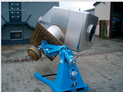
Pharmazeutischer Mischbehälter, Werkstoff 1.4404
