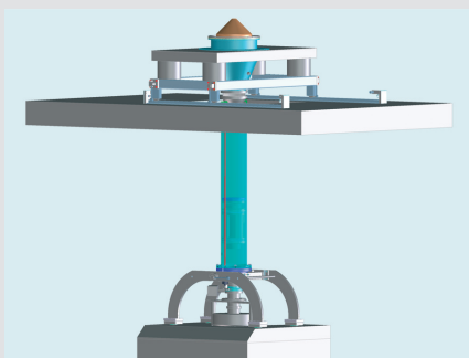
Befüllsystem VTS 200 aufgeständert auf einer Tabletten- presse
