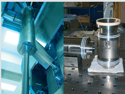
links: Füllsystem am Coater montiert rechts: Füllkopf in Edelstahl und Titan
